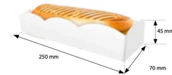
TR-109 Tacka na frytki, kurczaka, sałatki, gofry, itp. 250x70x45 mm Karton GC2, GC4 lub CKB
