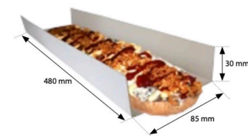
Z-102 Tacki idealne na zapiekanki, kanapki, gofry, itp. 480x85x30 mm Karton GC2, GC4 lub CKB
