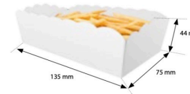
TR-102 Tacka klejona przestrzennie na frytki, kurczaka, sałatki, gofry, itp. 135x75x44 mm Karton GC2, GC4 lub CKB
